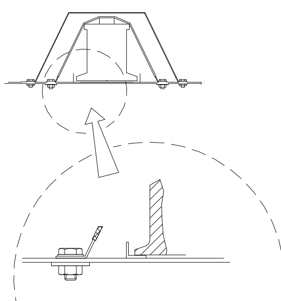
TEKENING 255-11
